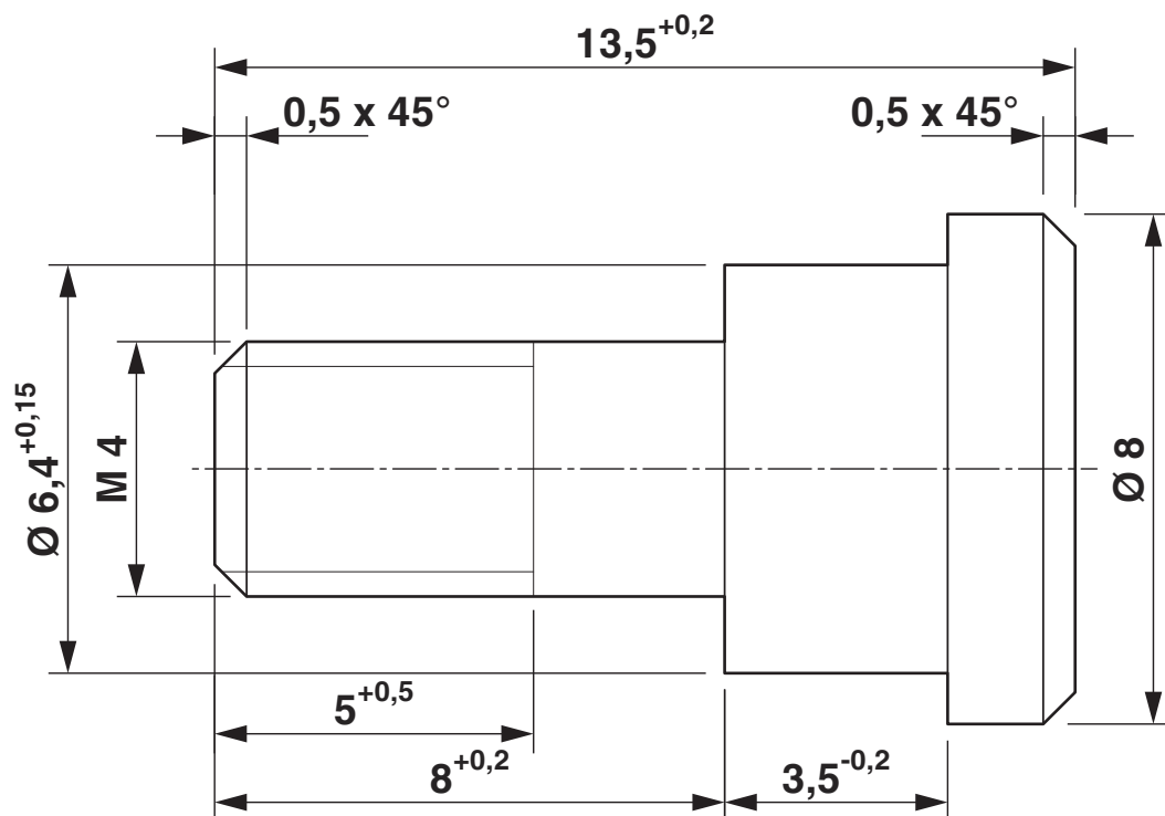
Maßzeichnung
