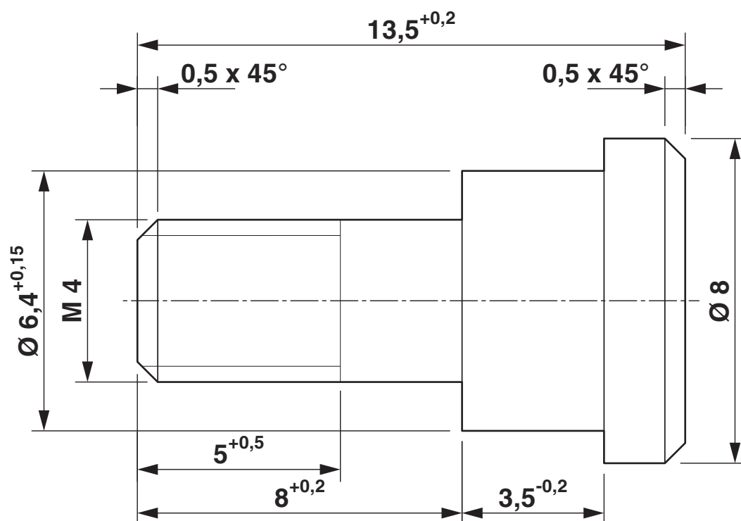
Dessin coté
