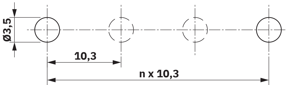
Maßzeichnung
