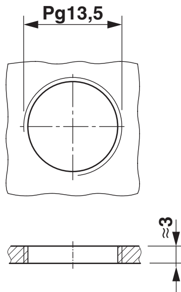
Maßzeichnung
