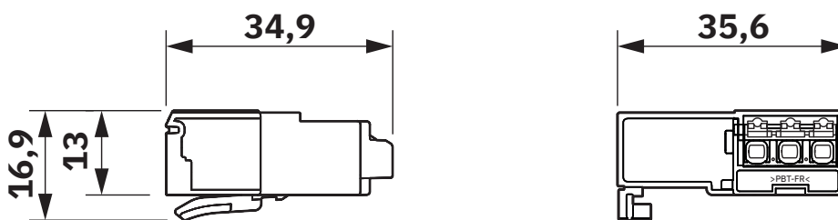
Dessin coté
