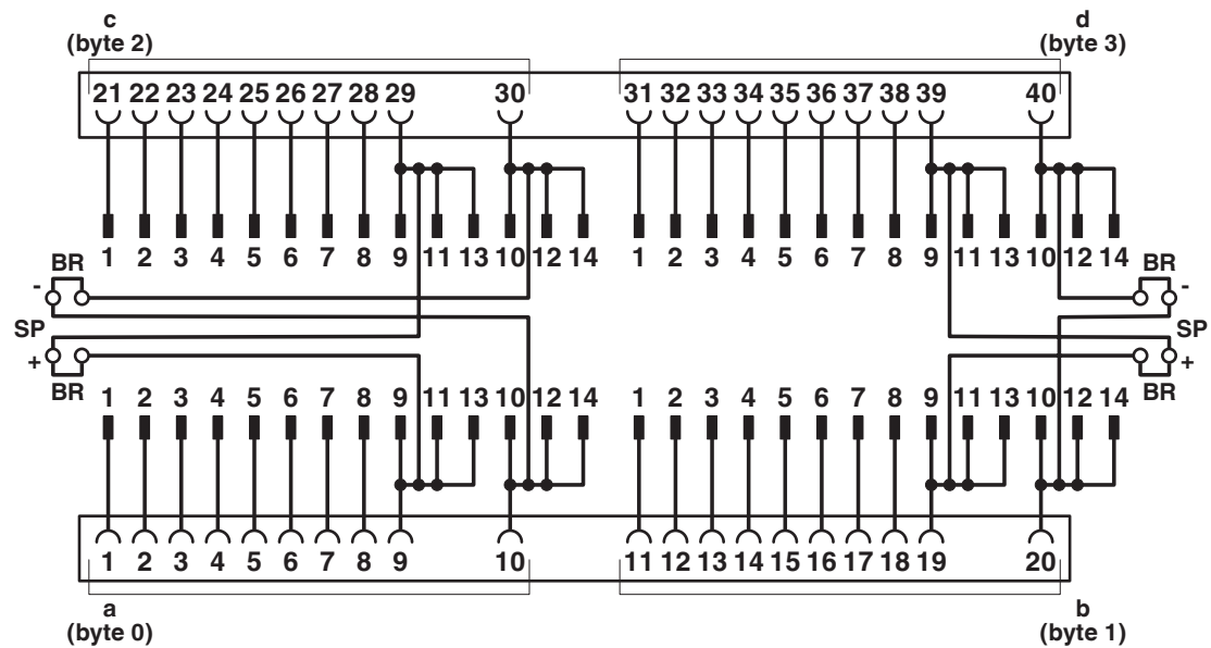
Anschlussbild FLKM 4X14-PA/.../DIO/S7-1500
