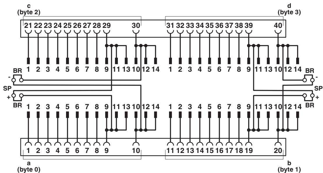
Esquema de conexiones FLKM 4X14-PA/.../DIO/S7-1500
