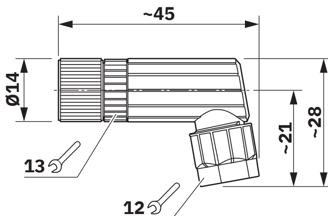
Maßzeichnung
