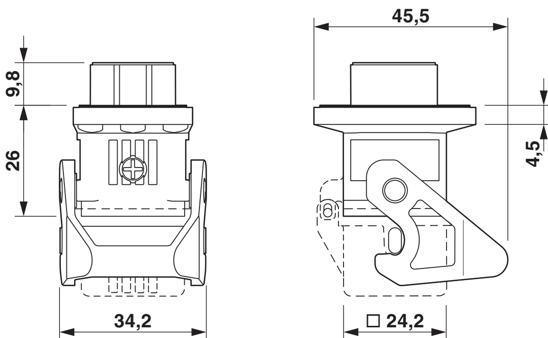
Dessin coté
