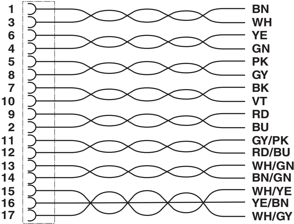
Diagrama eléctrico
