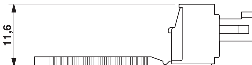
Esquema de dimensiones
