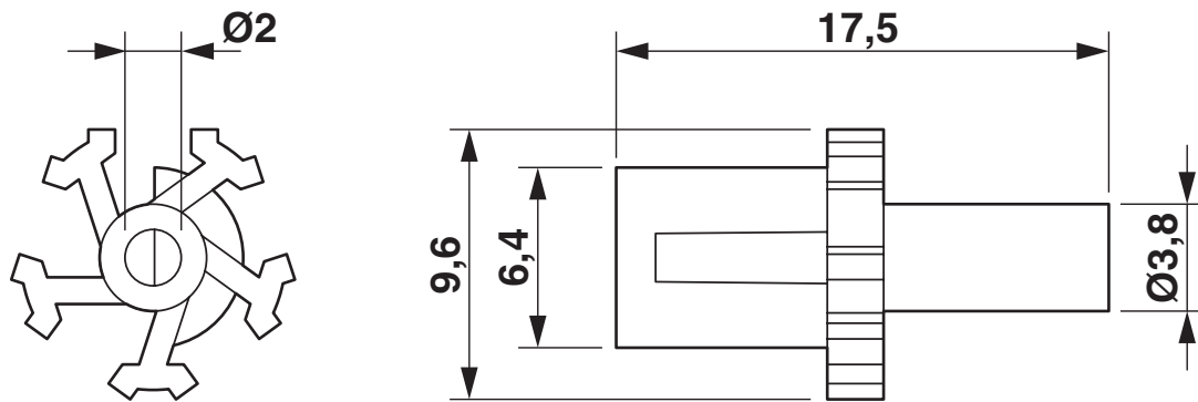
Maßzeichnung
