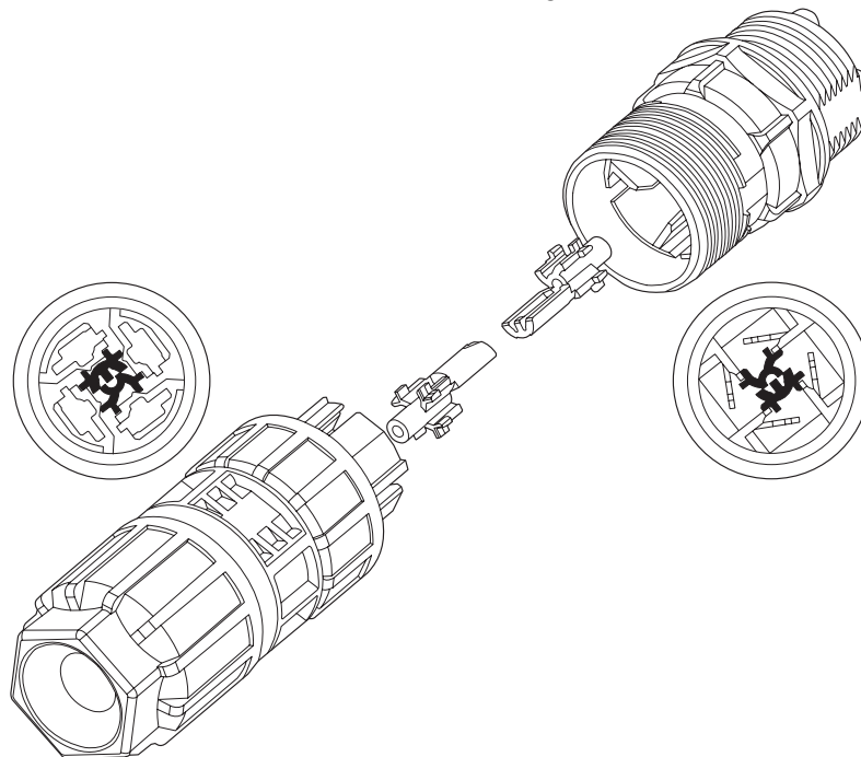
Schemazeichnung
