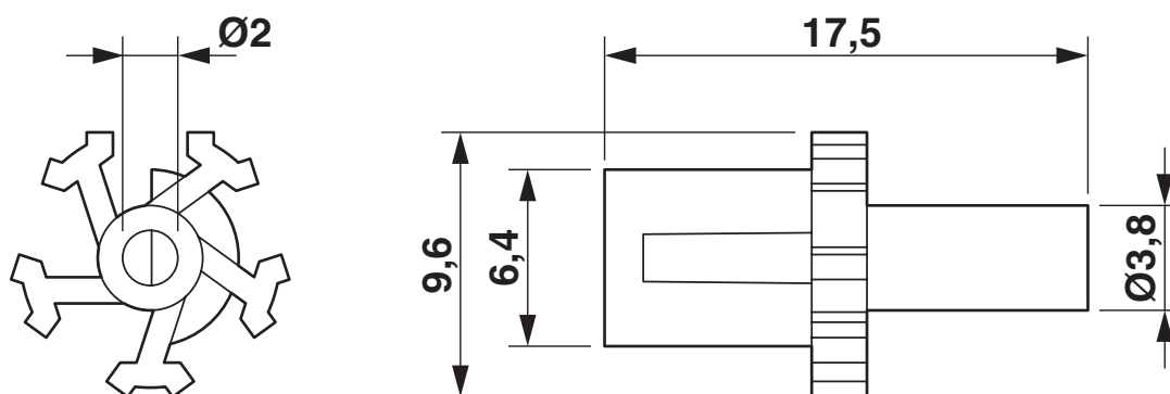
Dessin coté
