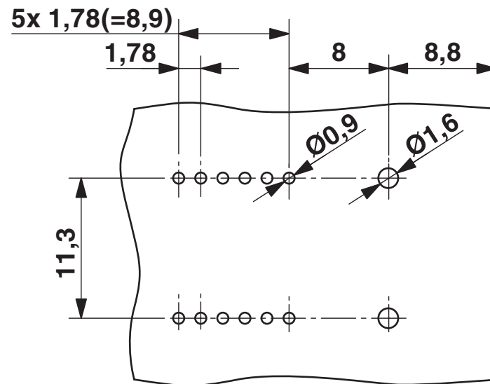
Bohrplan/Lötpadgeometrie
