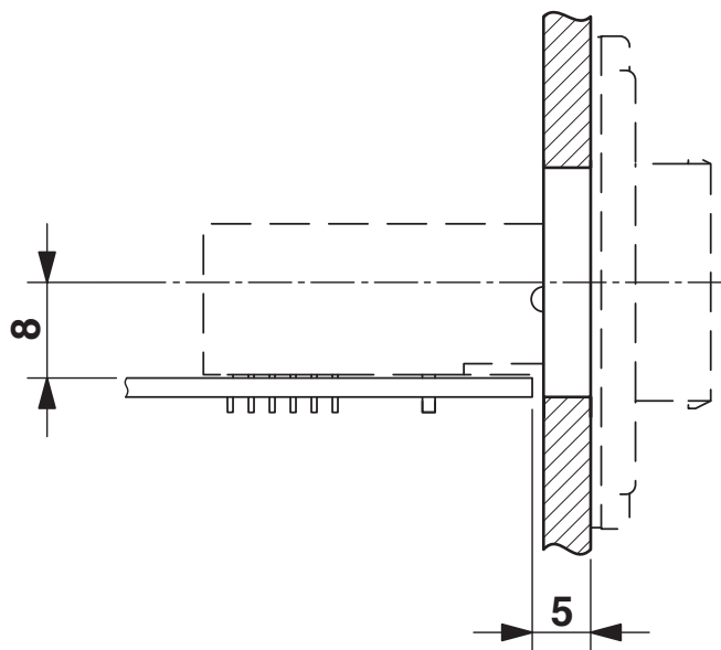
Dessin coté
