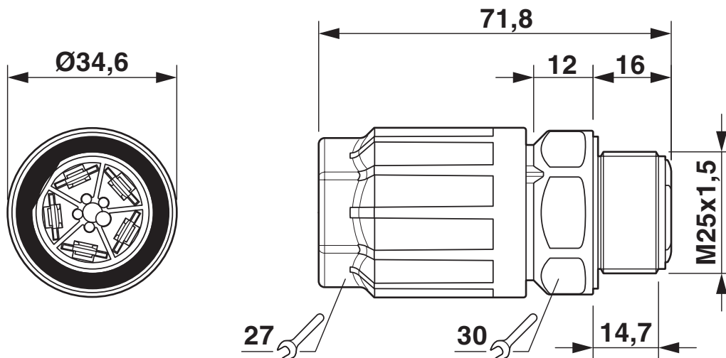
Dibujo acotado QPD W 4PE2,5 M25
