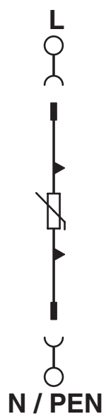
Diagrama eléctrico
