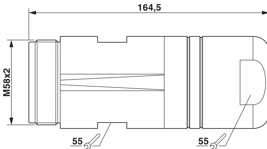
Maßzeichnung
