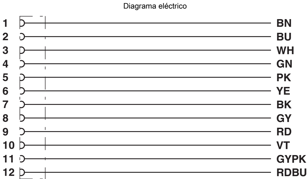
Ocupación de contactos del conector hembra M12
