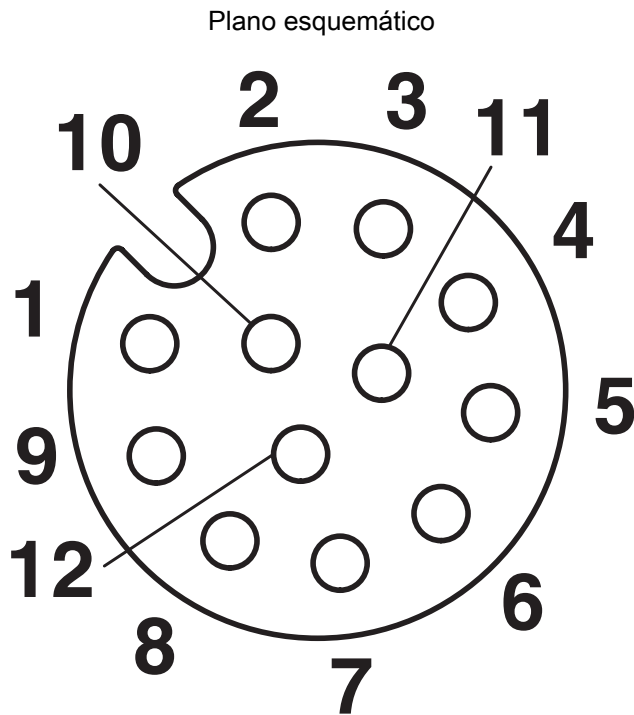
Esquema de polos del conector hembra M12, 12 polos, vista de la cara de hembras
