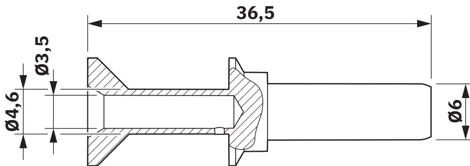
Dessin coté
