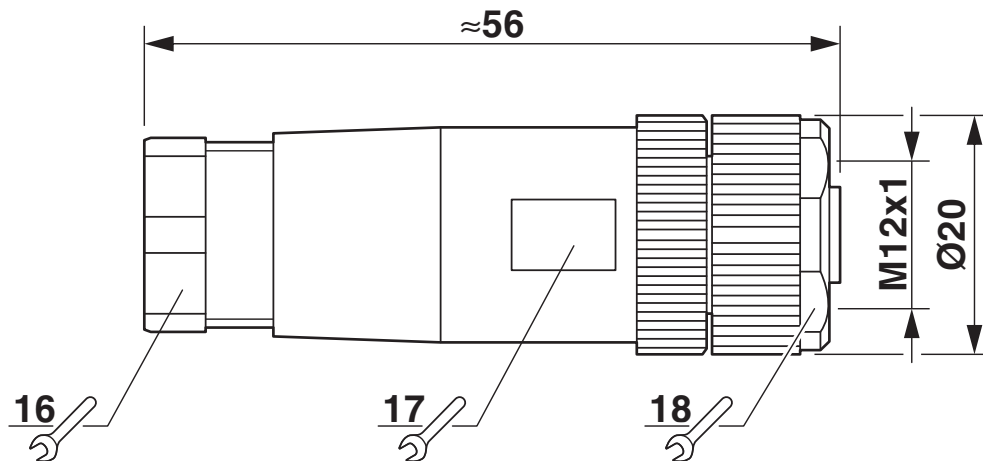
Maßzeichnung
