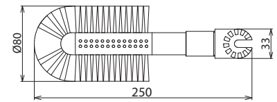
Maßbild STB 80 ZK MS
