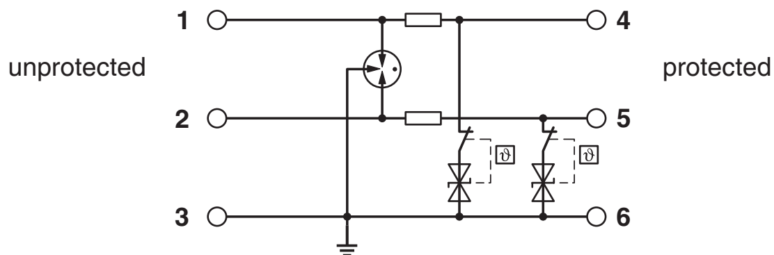
Diagrama eléctrico
