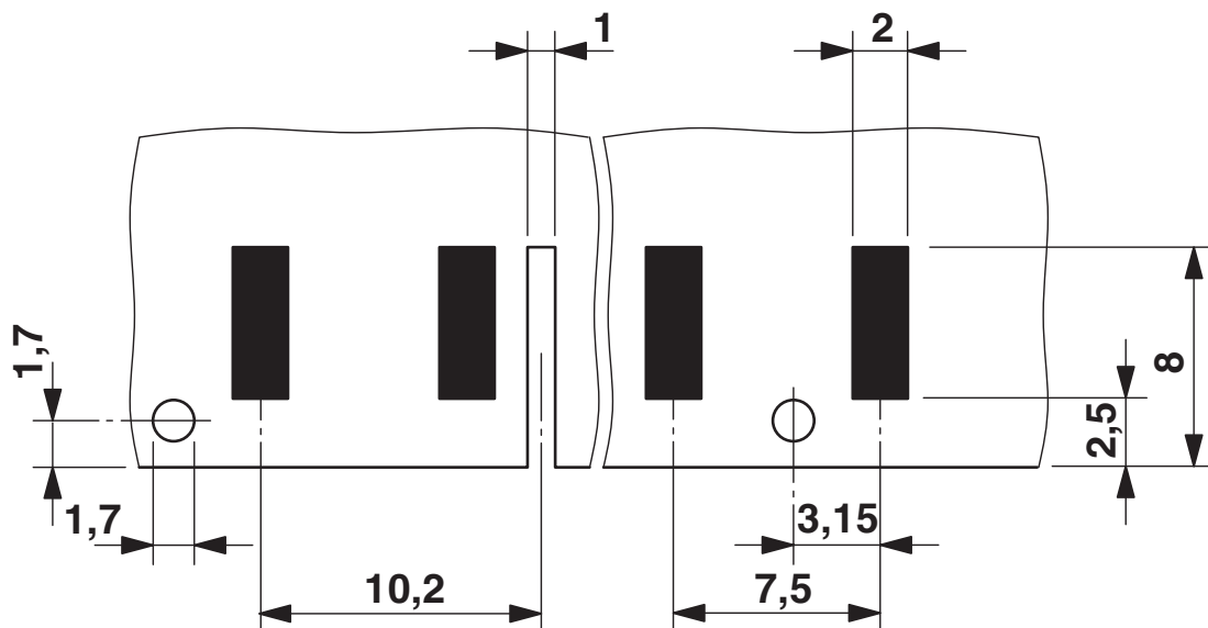
Bohrplan/Lötpadgeometrie
