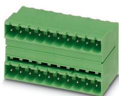
La figura muestra una variante de 10 polos con 20 contactos
