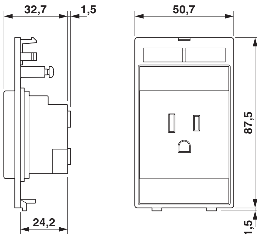
Dessin coté
