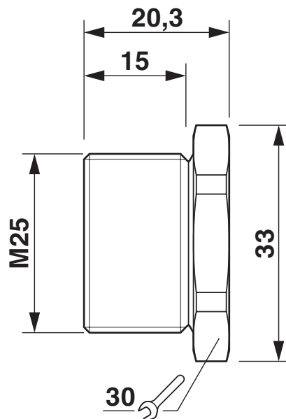
Maßzeichnung
