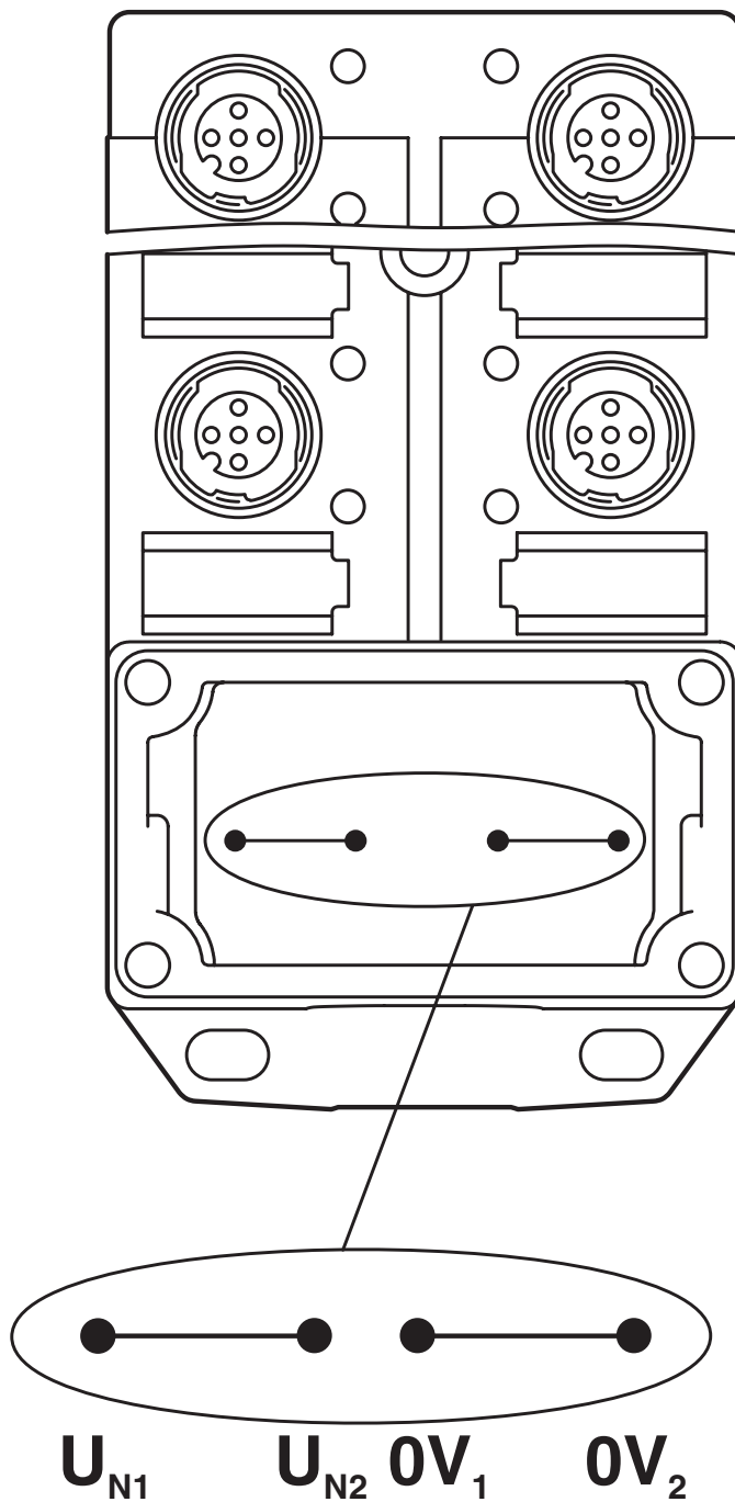
Plano esquemático
