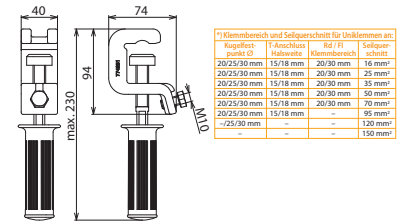
Maßbild UK K25 FL30 HG
