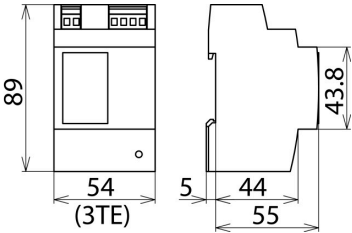
Dimensioni PSU DC24 30W
