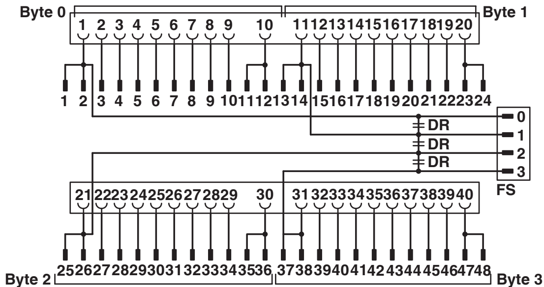
Anschlussbild FLKM 50-PA-S300
