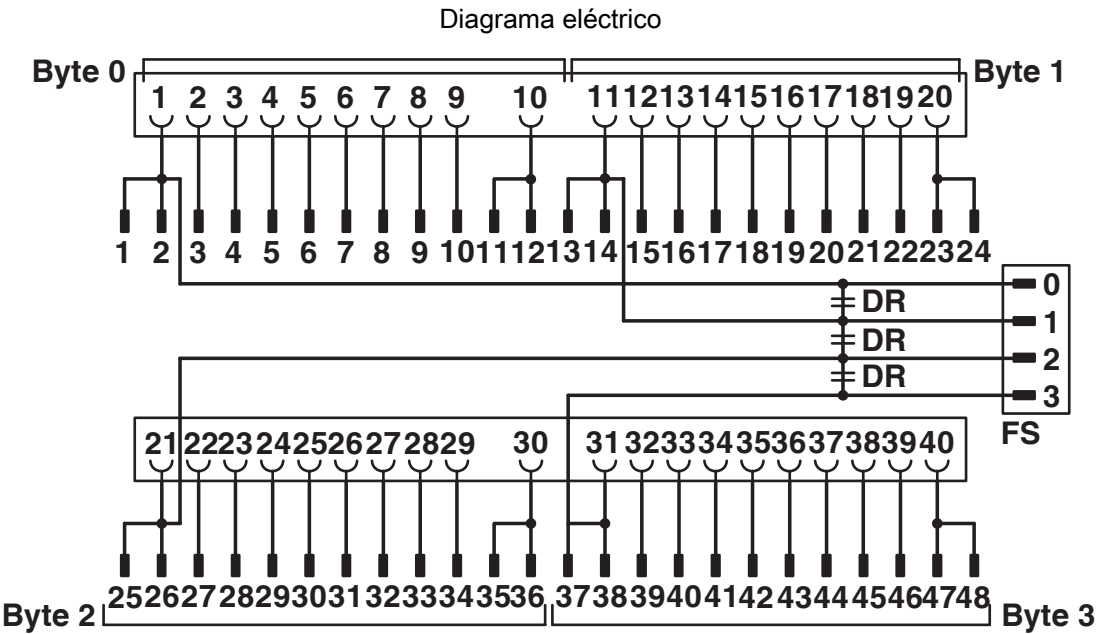
Esquema de conexiones FLKM 50-PA-S300
