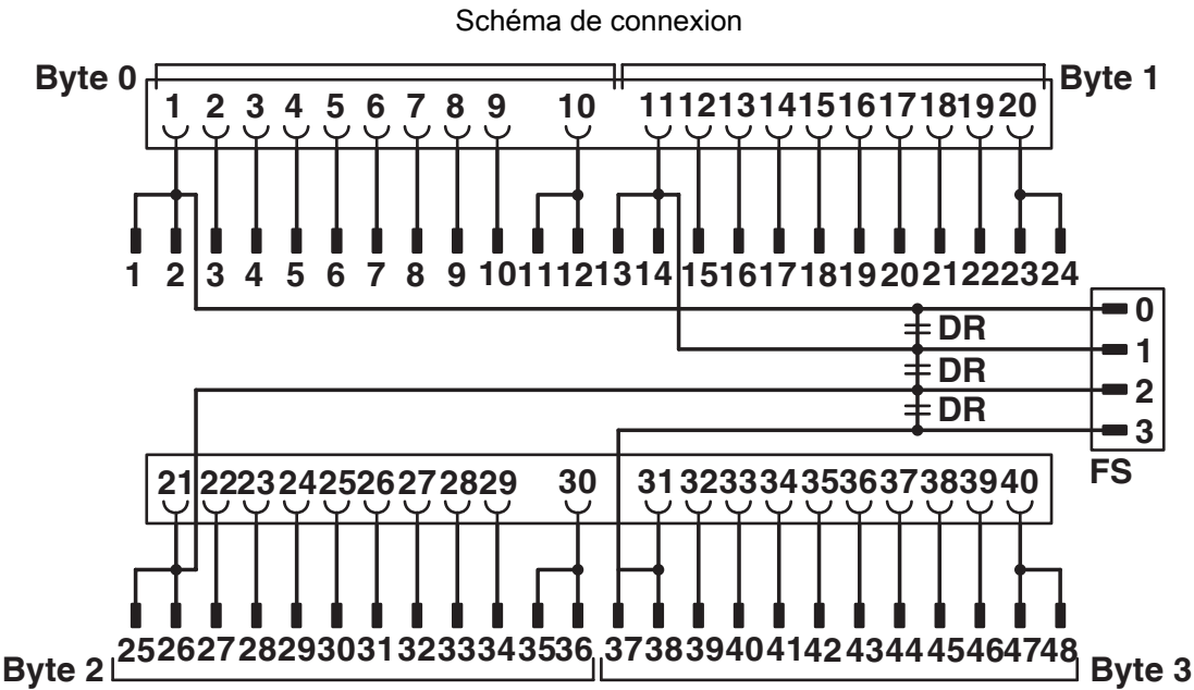
Schéma des connexions FLKM 50-PA-S300
