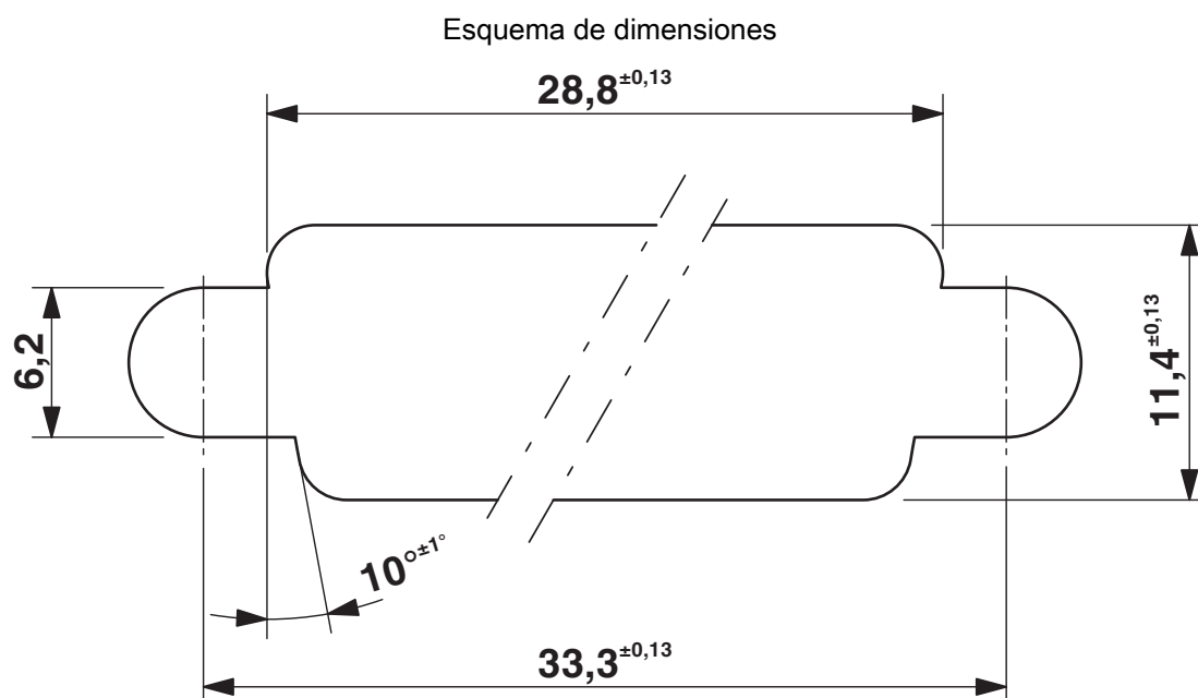
Plano esquemático
