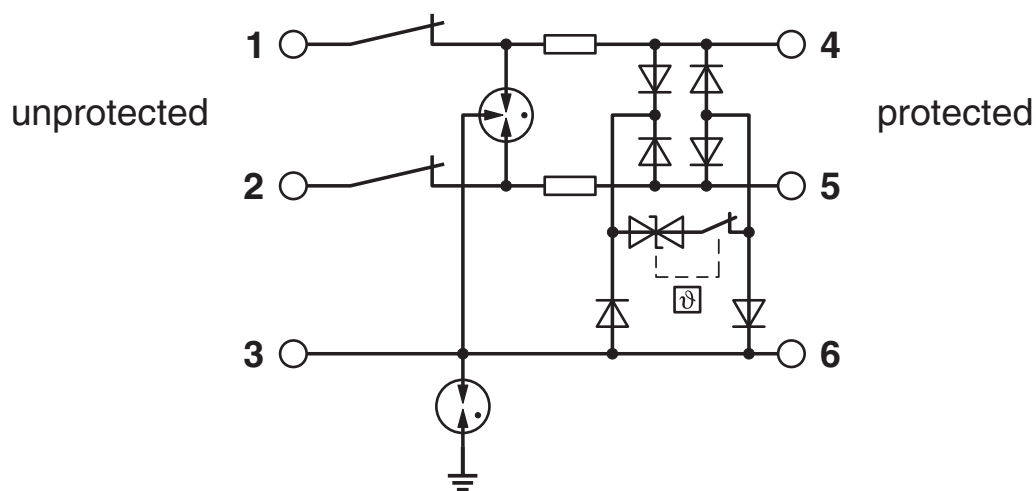
Schaltplan
