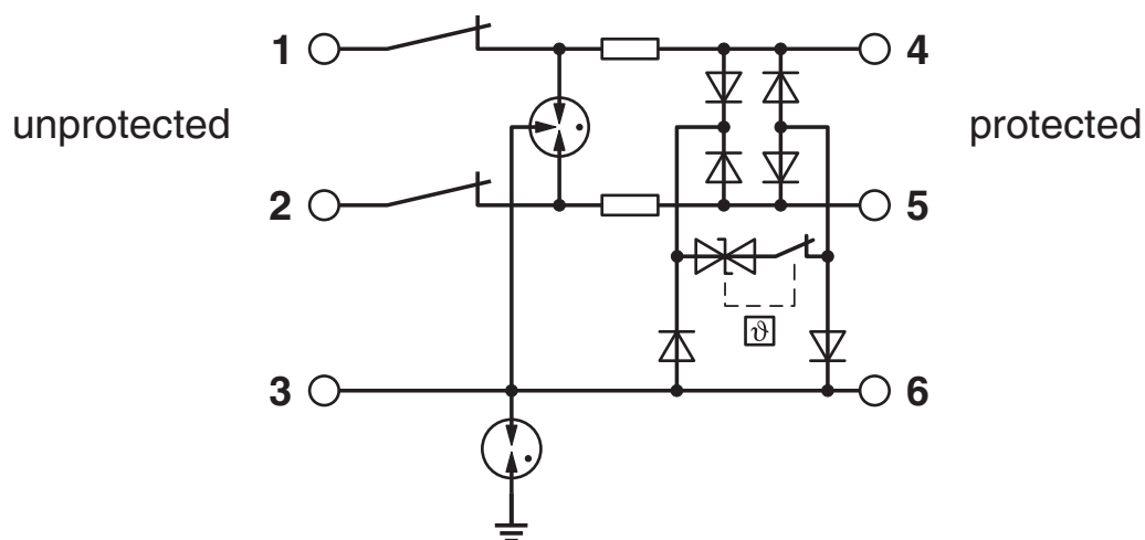
Diagrama eléctrico
