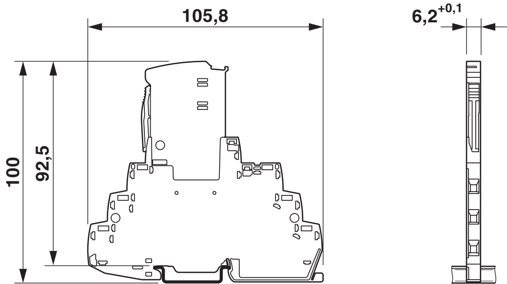
Plano esquemático
