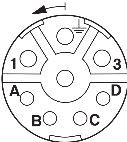
Plano esquemático
