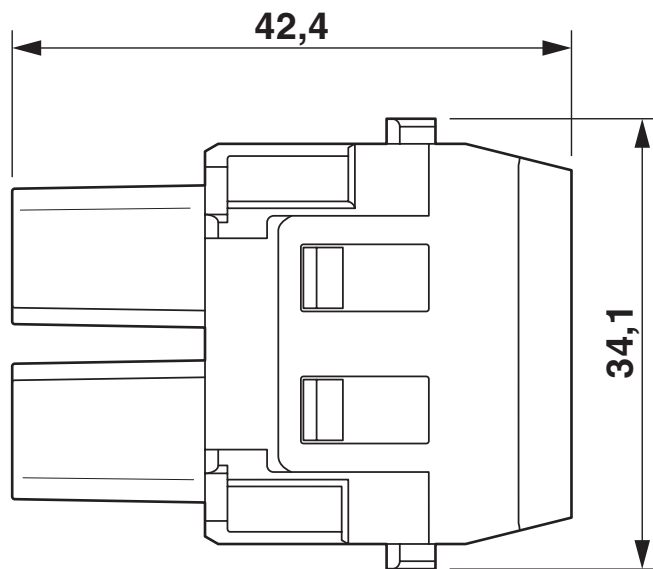
Maßzeichnung
