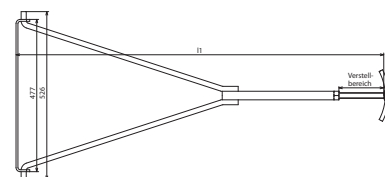
Maßbild TS 7.10 V1.0 1.15M STTZN
