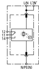
Esquema del DB M 1 320 FM
