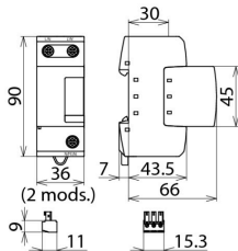
Dimensiones del DB M 1 320 FM
