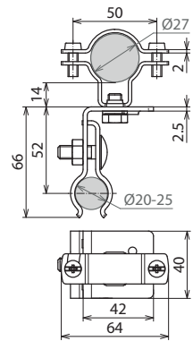
Maßbild DLH RSF ZS 27 V2A
