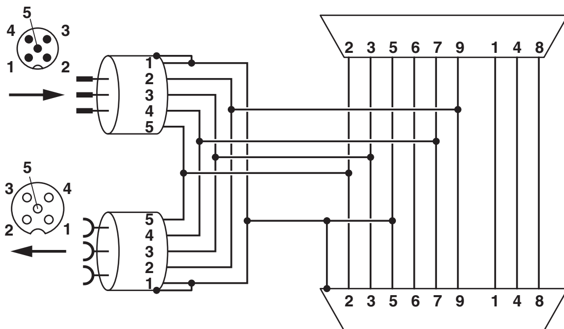
Diagrama de contactos de función SUBCON-PLUS-CAN/...M12
