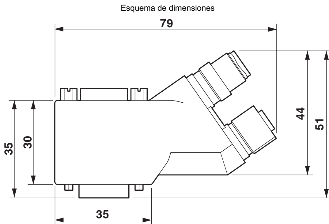
Esquema de dimensiones SUBCON-PLUS...35...M12, variante de 35°
