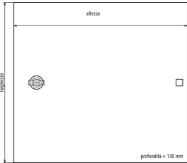
Dimensioni DPG LSA 120 P
