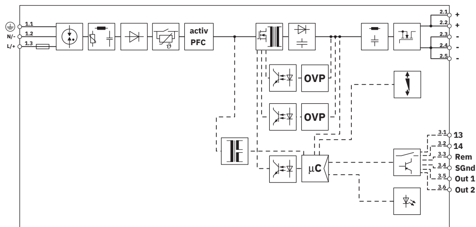
Schéma fonctionnel
