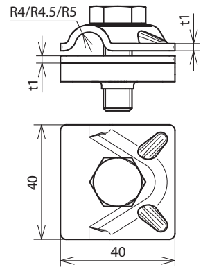
Maßbild MVK 10 SKM10X35 V2A
