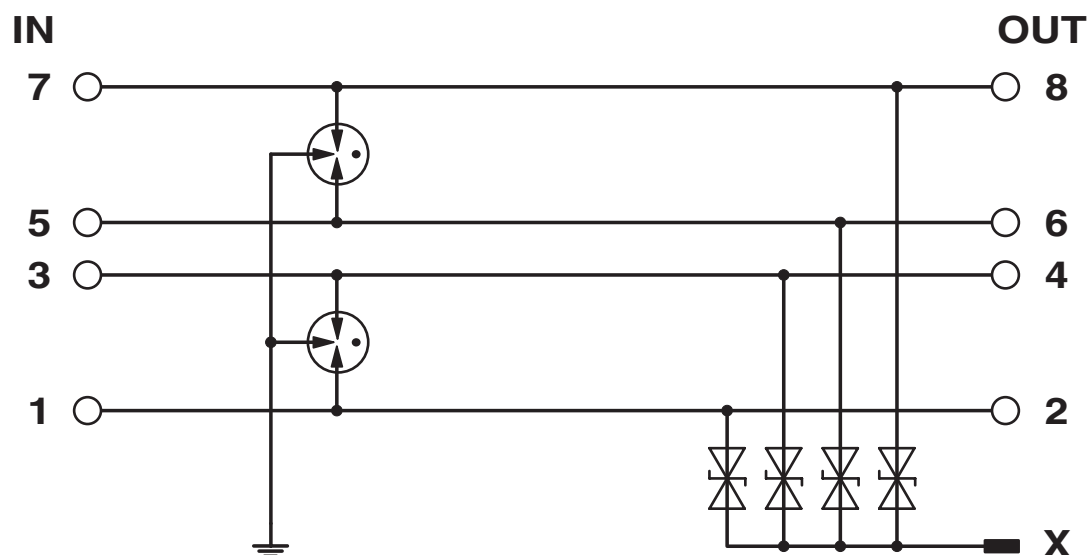
Diagrama eléctrico
