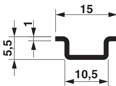
Dessin coté
