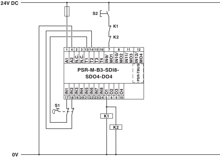
Applikationszeichnung
