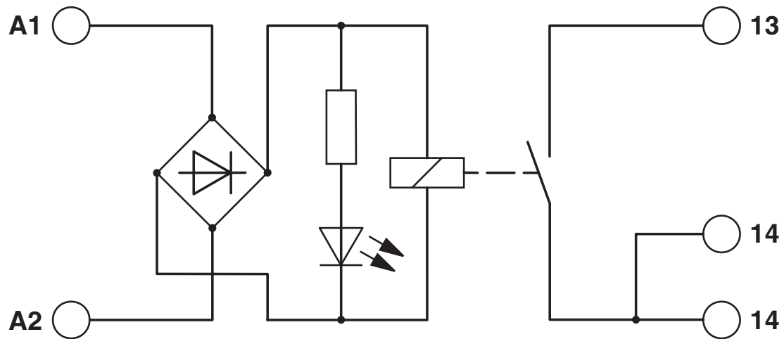
Diagrama eléctrico
