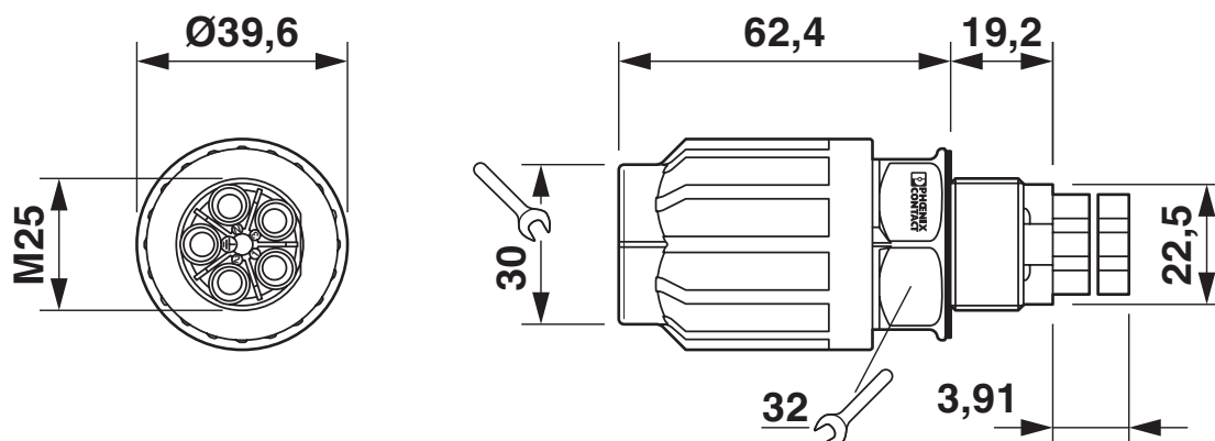
Dibujo acotado QPD W 4PE6,0 M25
